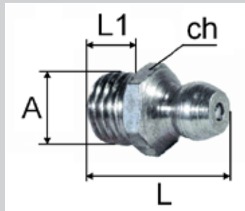
Fettpresse HYDRAULIK gerade mit Kugelkopf. Gemäß Norm UNI 7.663 A
